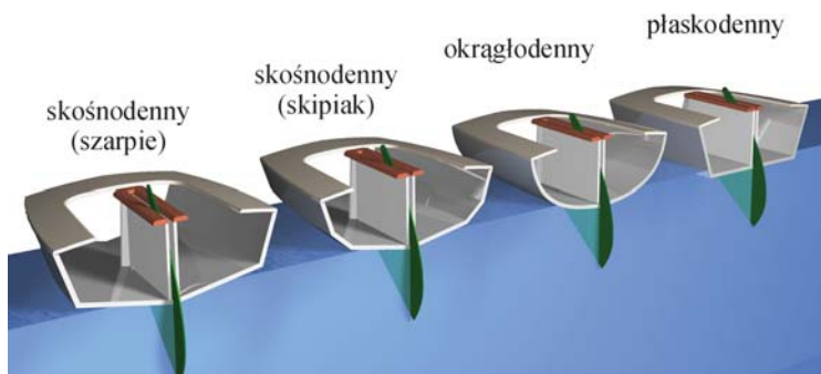
Rys. 3.5. Przekroje poprzeczne kadłuba jachtu mieczowego
