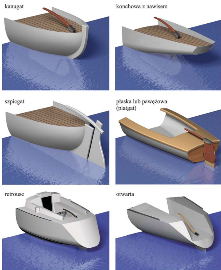
Rys. 3.6. Rodzaje rozwiązań rufy jachtu
